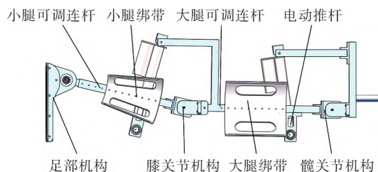
图 1 下肢康复机器人外骨骼结构
